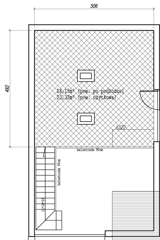
RZUT ANTRESOLI
