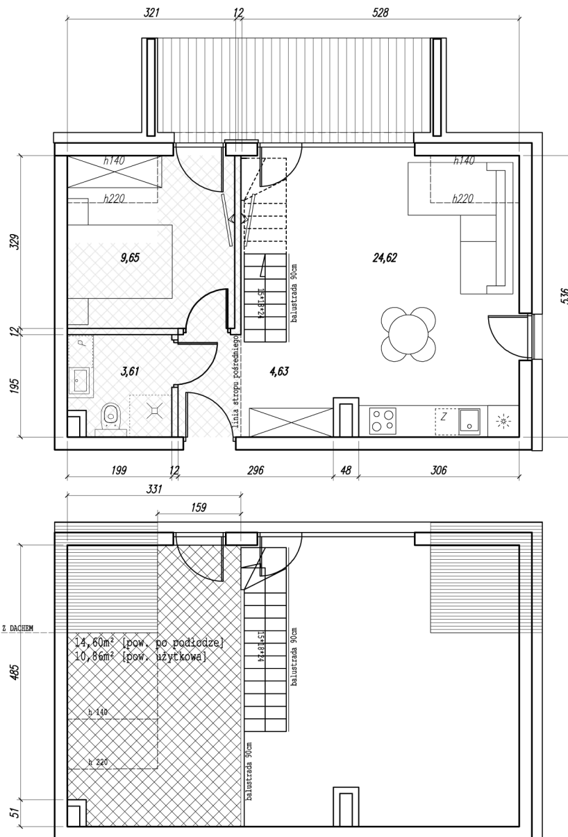
RZUT ANTRESOLI
